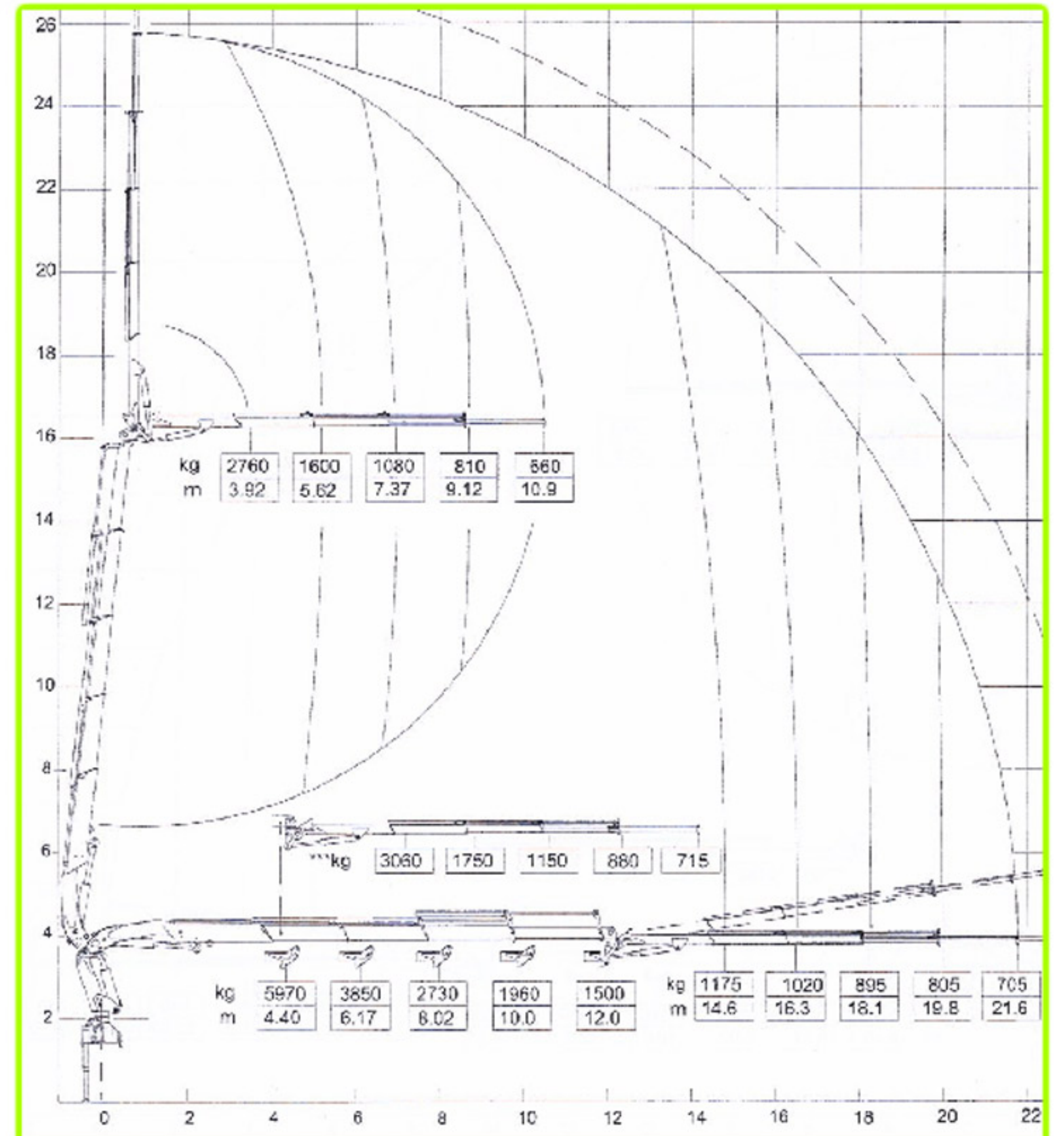
Lastdiagram met Jib
