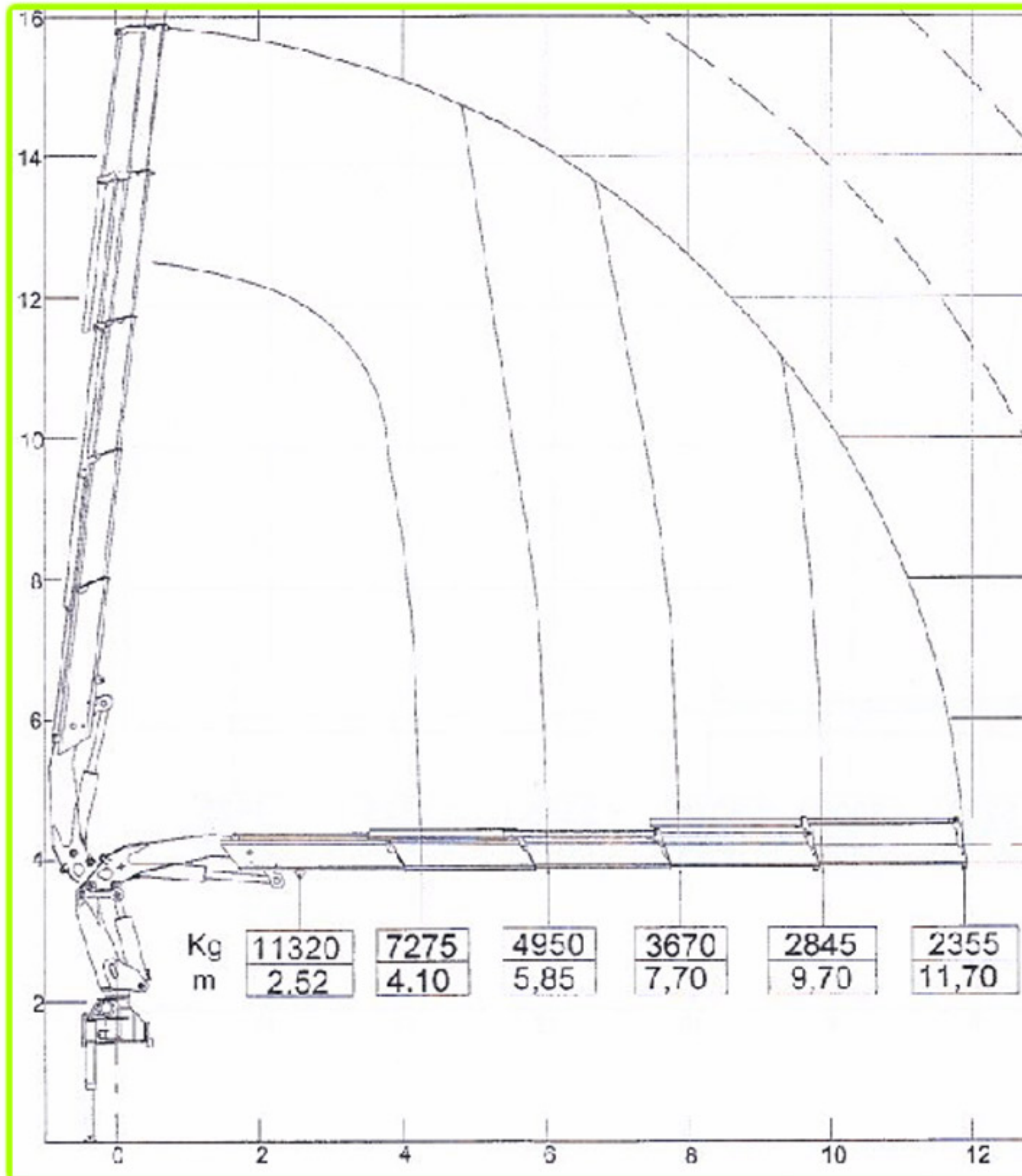
Lastdiagram zonder Jib
